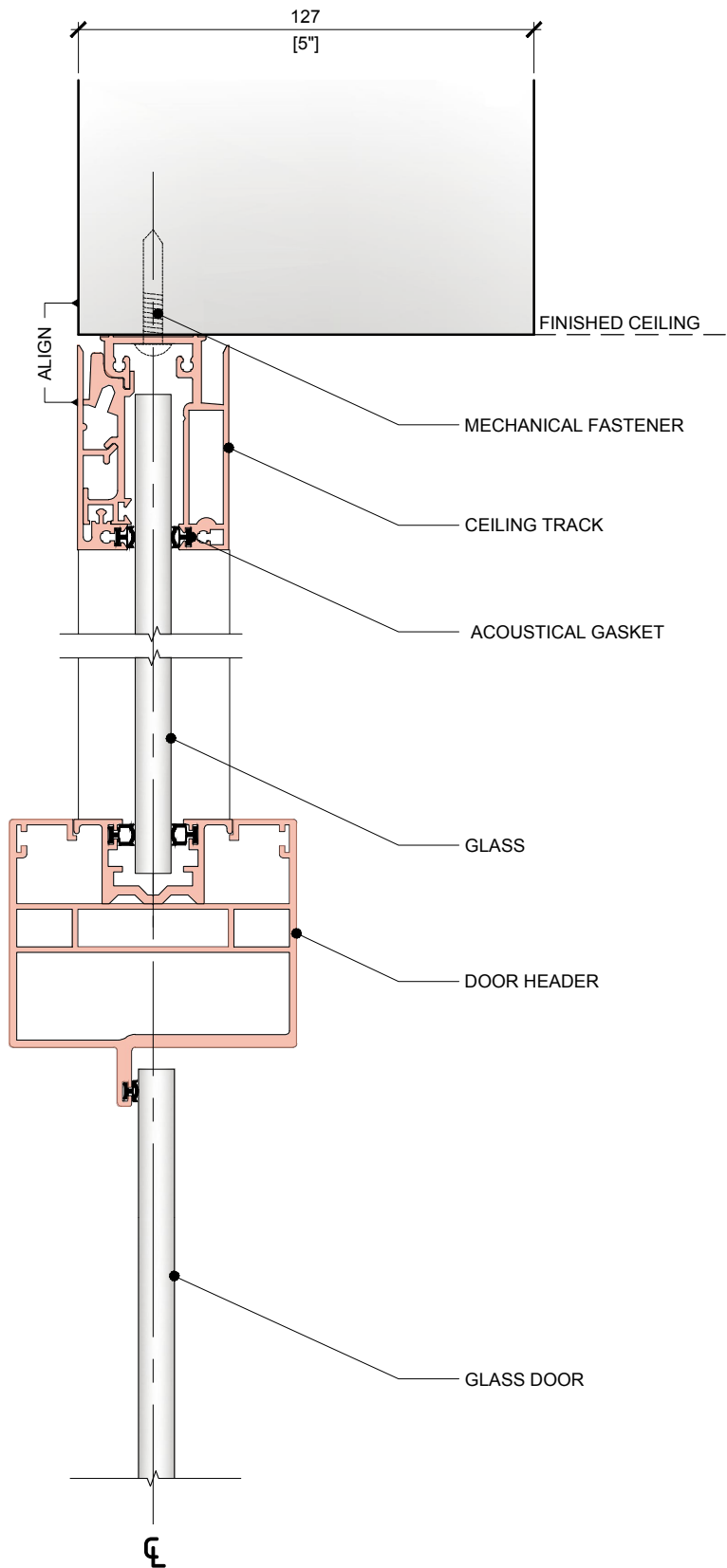
01 DWEL: GLASS HINGED DOOR - C/W TRANSOM D18 1:2
