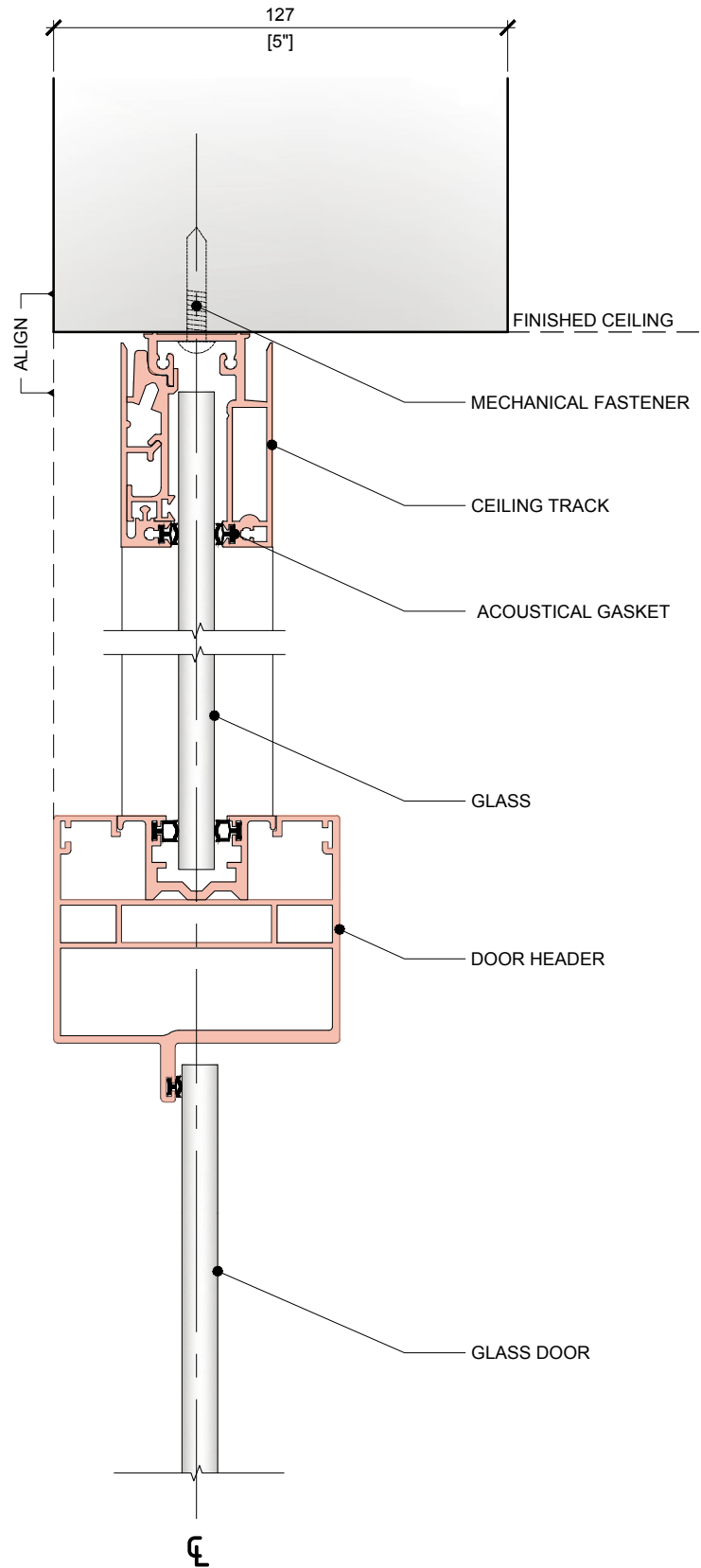
01 DWEL: GLASS HINGED DOOR - C/W TRANSOM D19 1:2
