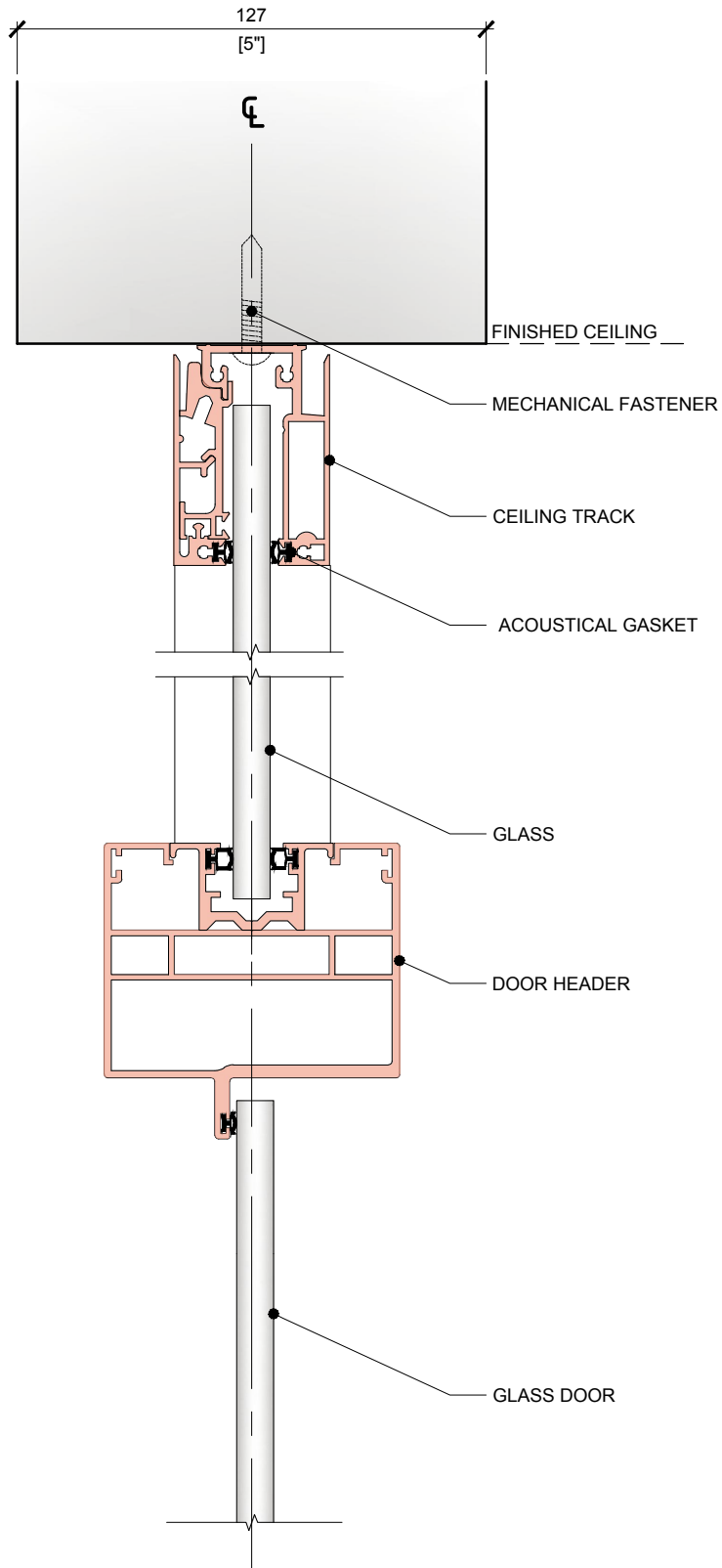
01 DWEL: GLASS HINGED DOOR - C/W TRANSOM D24 1:2
