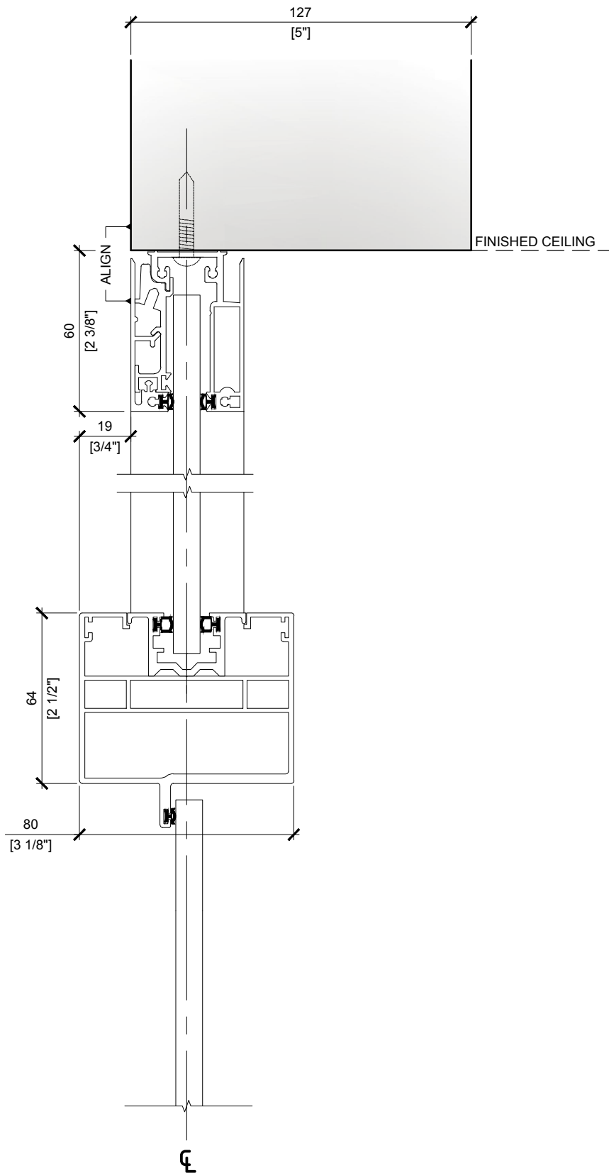
01 DWEL: GLASS HINGED DOOR - C/W TRANSOM - DIM DM18 1:2
