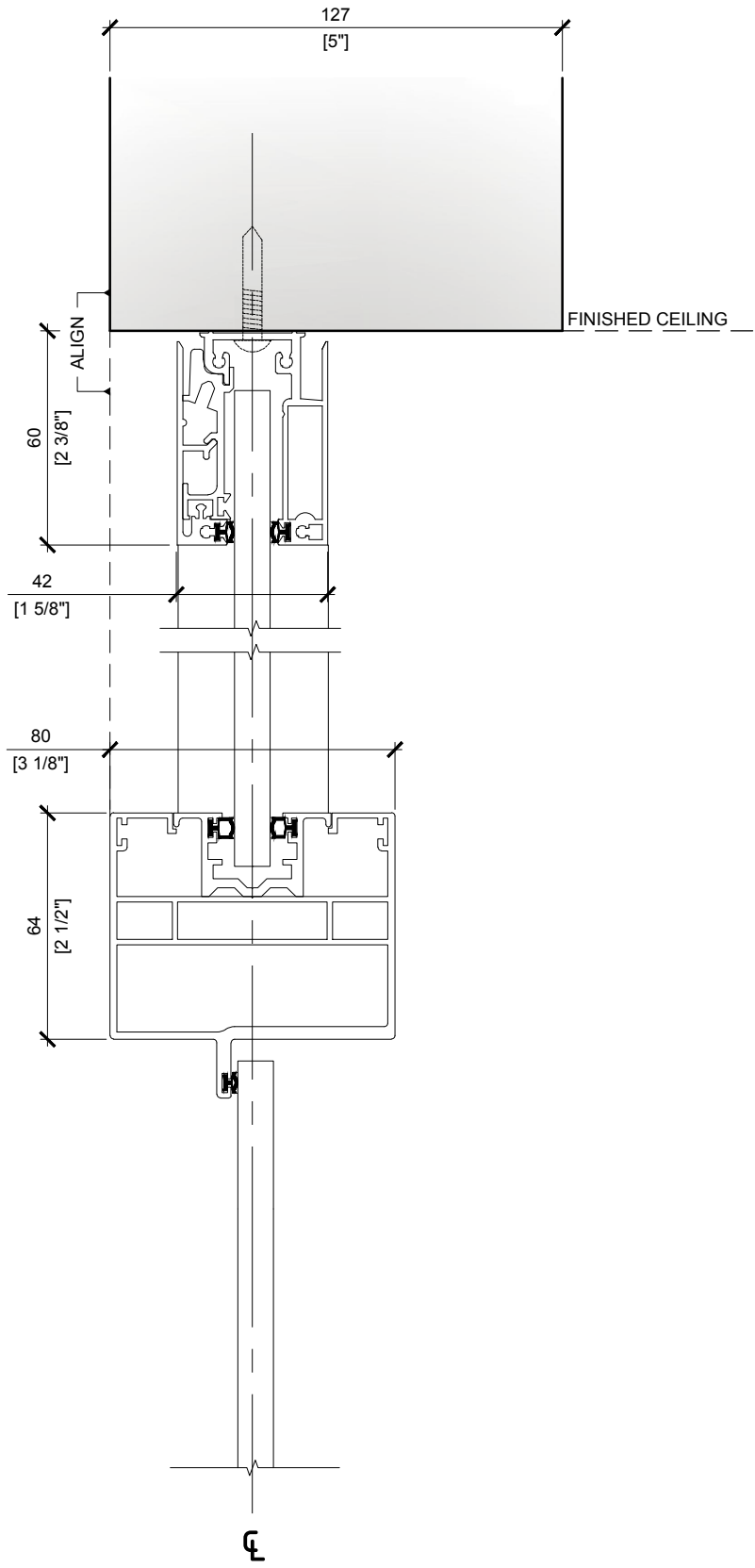
01 DWEL: GLASS HINGED DOOR - C/W TRANSOM - DIM DM19 1:2
