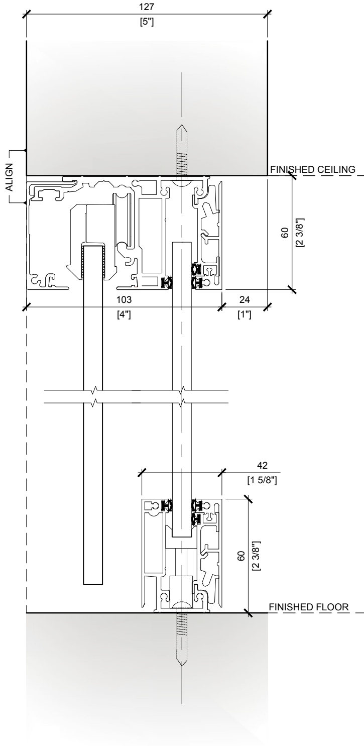
01 DWEL: GLASS SLIDING DOOR - DIM DM21 1:2
