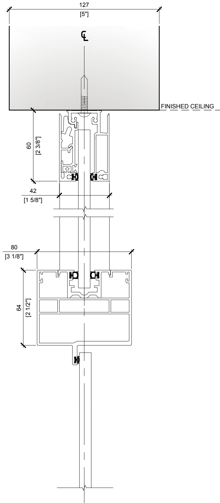
01 DWEL: GLASS HINGED DOOR - C/W TRANSOM - DIM DM24 1:2
