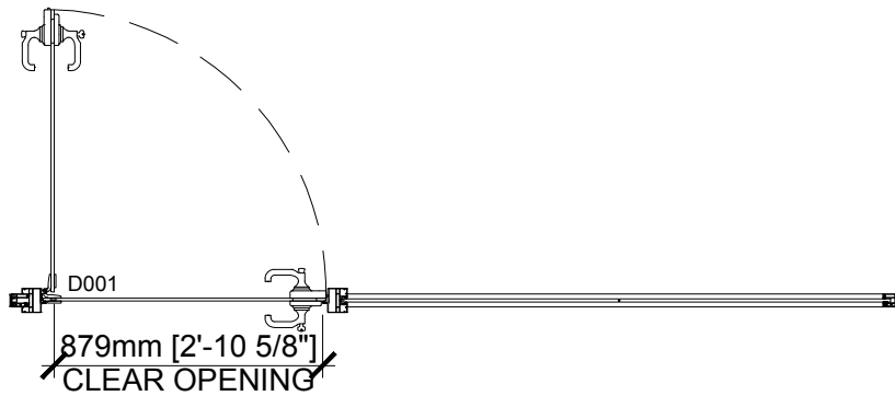
01 DWEL: GLASS HINGED DOOR - FULL HEIGHT E106 NTS
