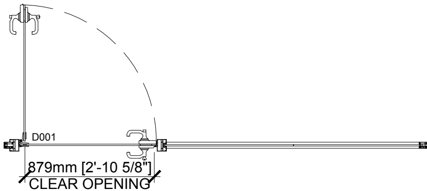
01 DWEL: GLASS HINGED DOOR - FULL HEIGHT E107 NTS
