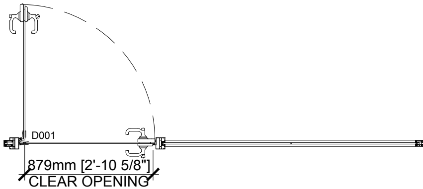
01 DWEL: GLASS HINGED DOOR - C/W TRANSOM E108 NTS
