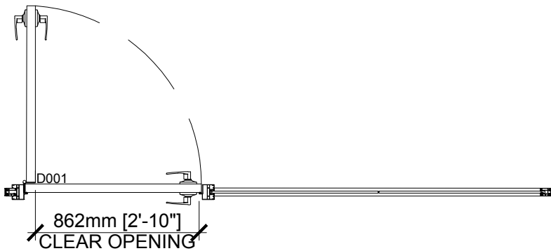
01 DWEL: WOOD HINGED DOOR - FULL HEIGHT E109 NTS
