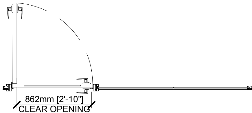
01 DWEL: WOOD DOOR WITH GLASS INSERT - C/W TRANSOM E112 NTS
