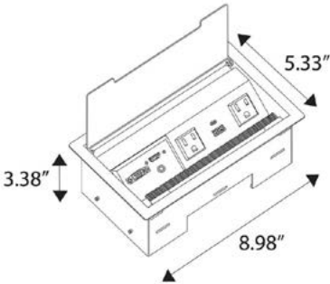
INTERACT G2
