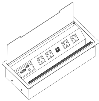
INTERFACE G2
