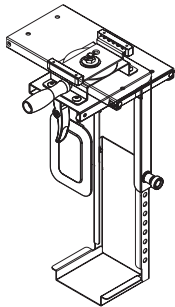
MINI SLIDE AND SWIVEL
